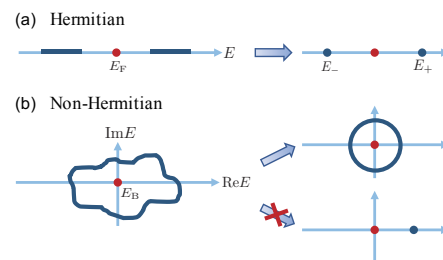
図：非エルミート系において現れる新たなトポロジカル相。エルミート系では絶縁体は実軸上のバンドギャップによって特徴づけられるが [(a)]、非エルミート系ではエネルギーが複素数となるため、バンド構造がある点 E_B の周りに巻き付くトポロジカル構造が可能となる [(b)]。Phys. Rev. X 8 , 031079 (2018) より転載。Phys. Rev. X 9 , 041015 (2019) も参照されたい。
