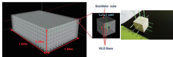
図 4. 新ニュートリノ検出器のひとつ、SuperFGD の概念図。 1 \times 1 \times 1 \text{ cm}^3 のプラスチックシンチレータ約 200 万個により、検出器内部で起きたニュートリノ反応の詳細な情報を捉える。
