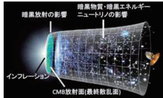
図 1: 宇宙進化の模式図。横軸が時間で、左側が宇宙初期、右が現在である。
