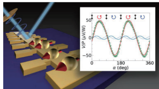
図 2. 光スピン変換現象の模式図と実験結果。
