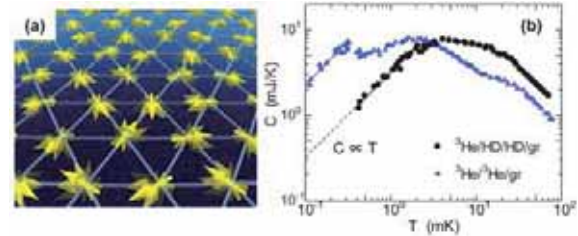
(a) 量子スピン液体のイメージ。(b) 2次元 ^3\text{He} C2相では、下地が ^3\text{He} 単原子層 ( \Delta ) と \text{HD}_2 分子層 ( \bullet ) の両方で、最低温度付近でギャップレスの量子スピン液体状態特有の温度に比例した熱容量が観測されています。
