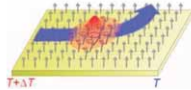
マグノンの熱ホール効果の概念図。(Science 329 , 297 (2010) より)
