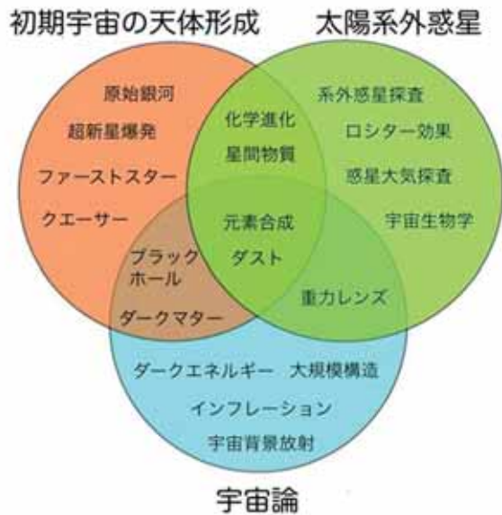
図1: 宇宙理論研究室で行われている研究テーマの概念図。3つの分野が有機的に結びついていることが分かる。
