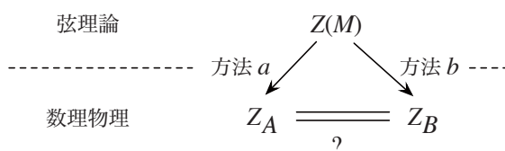
図 2: 弦理論からの「不思議な関係」の導出
