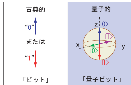
図：ベクトル表示での古典情報（ビット）と量子情報（量子ビット）との比較。ビットは上向き“0”または下向き“1”のいずれかのベクトルのみをとるが、量子ビットは上向き状態 |0\rangle と下向き状態 |1\rangle のみならず、これらの任意の量子力学的重ね合わせ状態をとることができるため、球面上どの向きのベクトルもとることができる。
