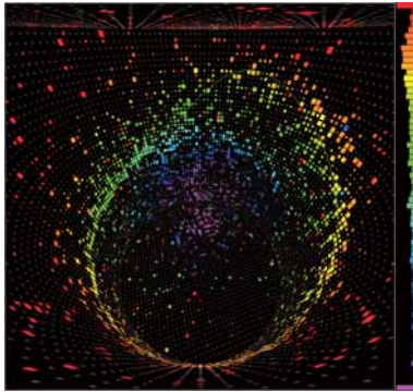
図 3. スーパーカミオカンデ検出器でとらえた、加速器ニュートリノビームによるニュートリノ反応事象。粒子が放つチェレンコフ光がリング状に見える。
