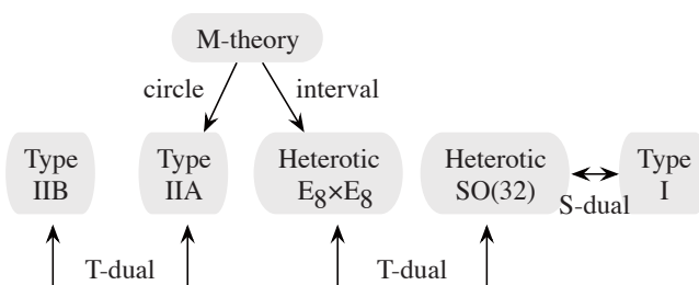
図 1: 超弦理論の双対性
