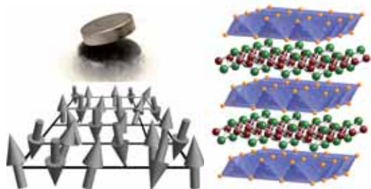
図1. 左：高温超伝導体が「ゲージ対称性の破れ」のために磁気浮上している様子と、高温超伝導体の理論的模型、矢印は電子スピン。右：最近我国で発見された鉄化合物高温超伝導体の結晶構造。
