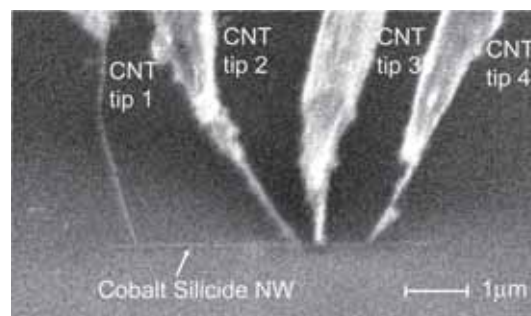
図2 : ミクロな針を使った4探針電気伝導測定
