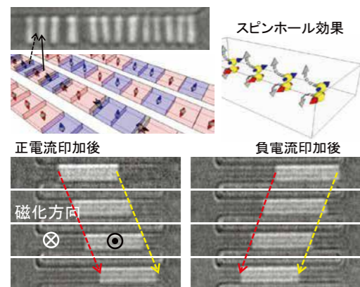
図1. カイラル磁区構造がスピンホール効果によって電流で平行移動の様子を磁気光学顕微鏡を用いて観察した様子。
