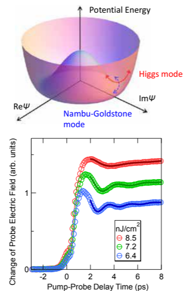
(上) 超伝導体の自由エネルギーを秩序変数の関数として示した模式図。動径方向の振動をヒッグスモードと呼ぶ。(下) 超伝導体 NbTiN で観測されたヒッグスモードの実時間観測。
