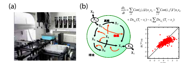
図(a) ラボオートメーションを用いた進化実験システムの外観。(b) 進化シミュレーションの一例。
