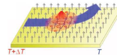
マグノンの熱ホール効果の概念図。(Onose et al. , Science 329 , 297 (2010) より。)
