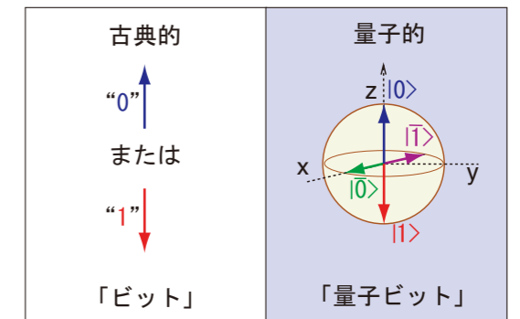
図：ベクトル表示での古典情報(ビット)と量子情報(量子ビット)との比較。ビットは上向き“0”または下向き“1”のいずれかのベクトルのみをとるが、量子ビットは上向き状態 |0\rangle と下向き状態 |1\rangle のみならず、これらの任意の量子力学的重ね合わせ状態をとることができるため、球面上どの向きのベクトルもとることができる。
