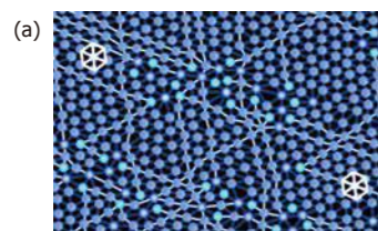
(a) 量子ヘキサティック相の概念図。
