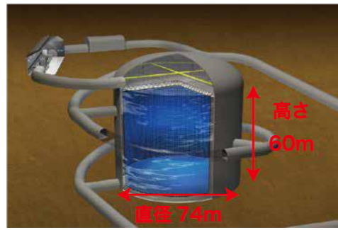
図4. ハイパーカミオカンデ検出器の概念図。高さ60m、直径74mのタンクに超純水を満たし、チェレンコフ光を検出することで多様な現象を捉える。
