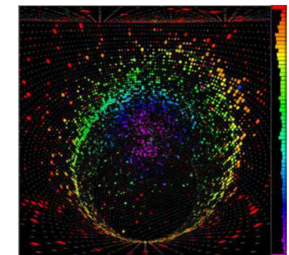
図 3. スーパーカミオカンデ検出器でとらえた、295km 離れた加速器からのニュートリノが反応した事象。チェレンコフ光がリング状に見える。
