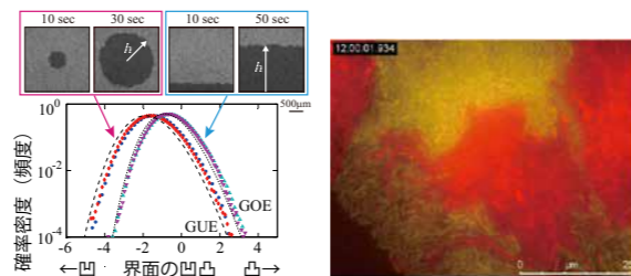
図1 (左)：液晶乱流の成長現象で発見した KPZ 普遍法則。界面の凹凸の分布が、普遍的な理論曲線に従っている。図2 (右)：均一環境で観察した、二種類の大腸菌集団の棲み分けの様子。
