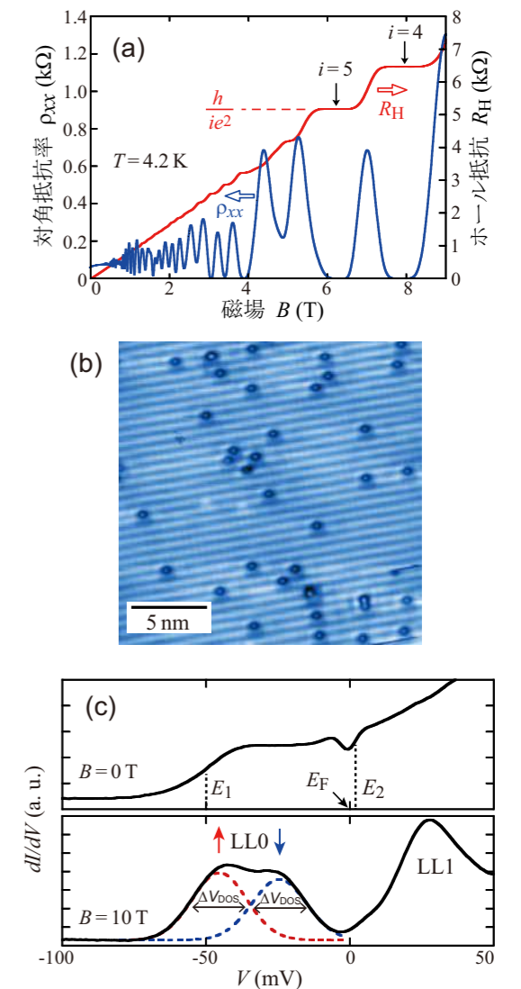
図1：(a) 二次元電子系における量子ホール効果。(b) STM 像。ランダムな黒丸が Fe 原子。(c) 同一試料で測定されたランダウ準位。
