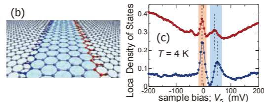
(b) スピン分極したz-GNRの概念図と(c)ジグザグ端上で測定した局所状態密度。(b)の左(右)端上のものを青(赤)色で示す。V s = 0, 50 mV付近のピークがスピン偏極状態に対応している。
