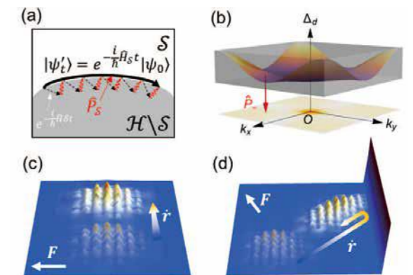
ゼノ・ホール効果。(a) 測定の反作用や散逸により、状態は特定の部分空間 S に拘束されながら、有効ハミルトニアン \hat{H}_S = \hat{P}_S \hat{H} \hat{P}_S により時間発展する。(b) 光格子中の冷却原子系に人工的に散逸を導入することで、波数空間中で粒子を非自明なペリ-曲率を持つ低エネルギー・バンドに拘束できる。このとき、粒子の実空間運動において、(c) ホール効果(外場 F の垂直方向への運動)および(d) 再帰性反射(入射方向への反射)が起きる。Phys. Rev. Lett. 118 , 200401 (2017) より転載。
