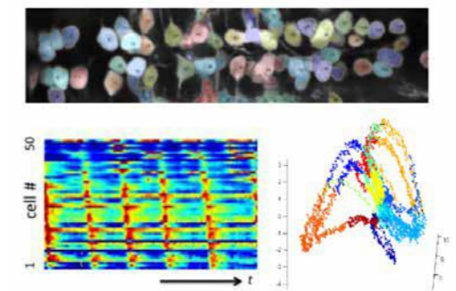
図1: カルシウムイメージングによる神経活動の解析。神経組織内の多数の細胞(上)の活動をイメージングデータから自動抽出し時間経過に伴う変化を系統的に解析する(左下、赤色が活動状態を示す)。クラスタリング解析や次元縮約により回路全体の状態変化を3次元空間内で可視化することもできる(右下)。
