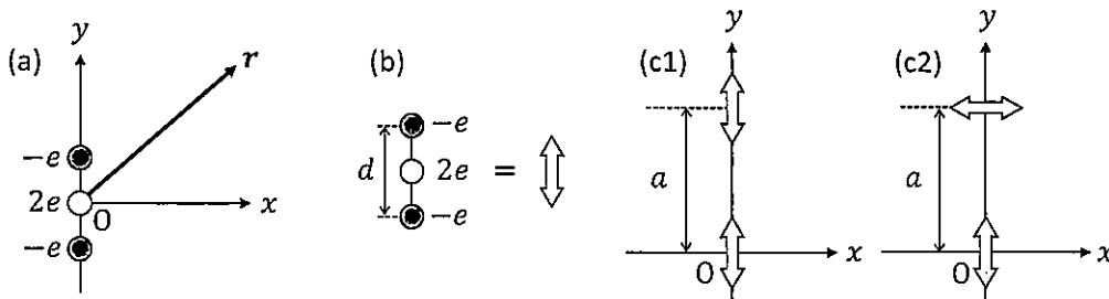
図 2: 電気四極子の配置図。
